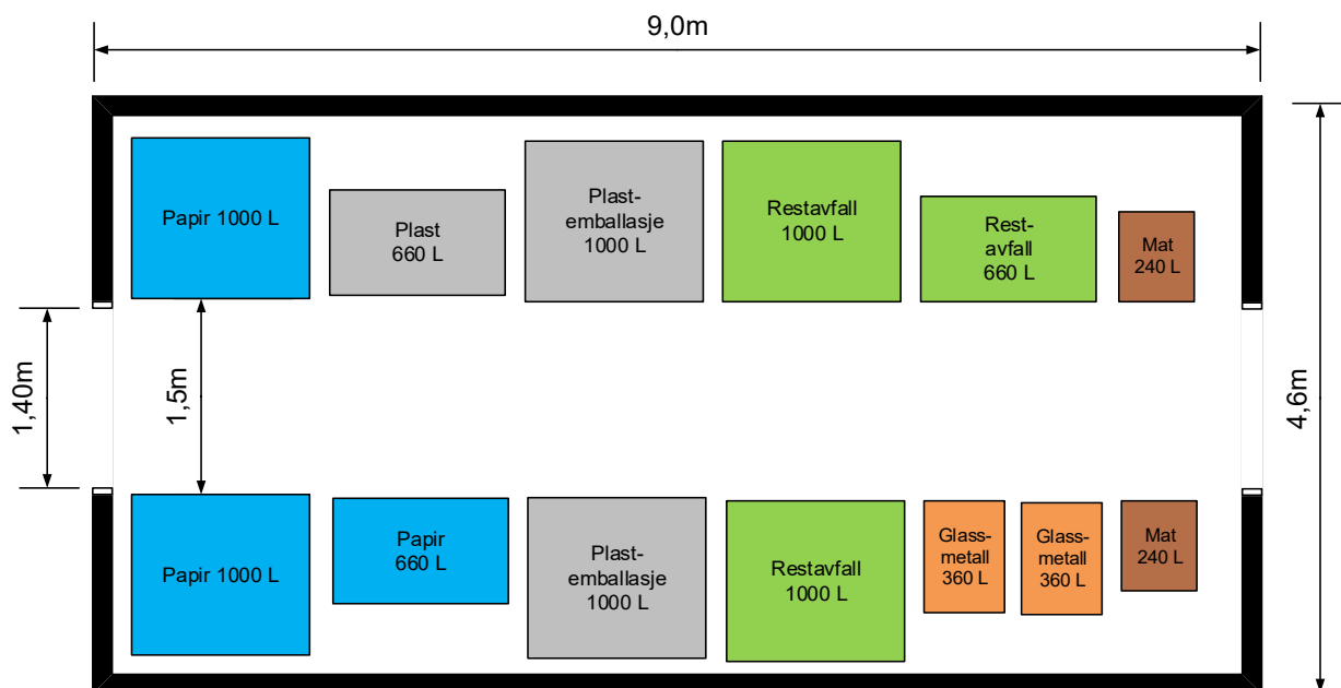
Figur 5-15: Eksempel på planløsning for avfallshus/avfallsrom for 20 husstander
