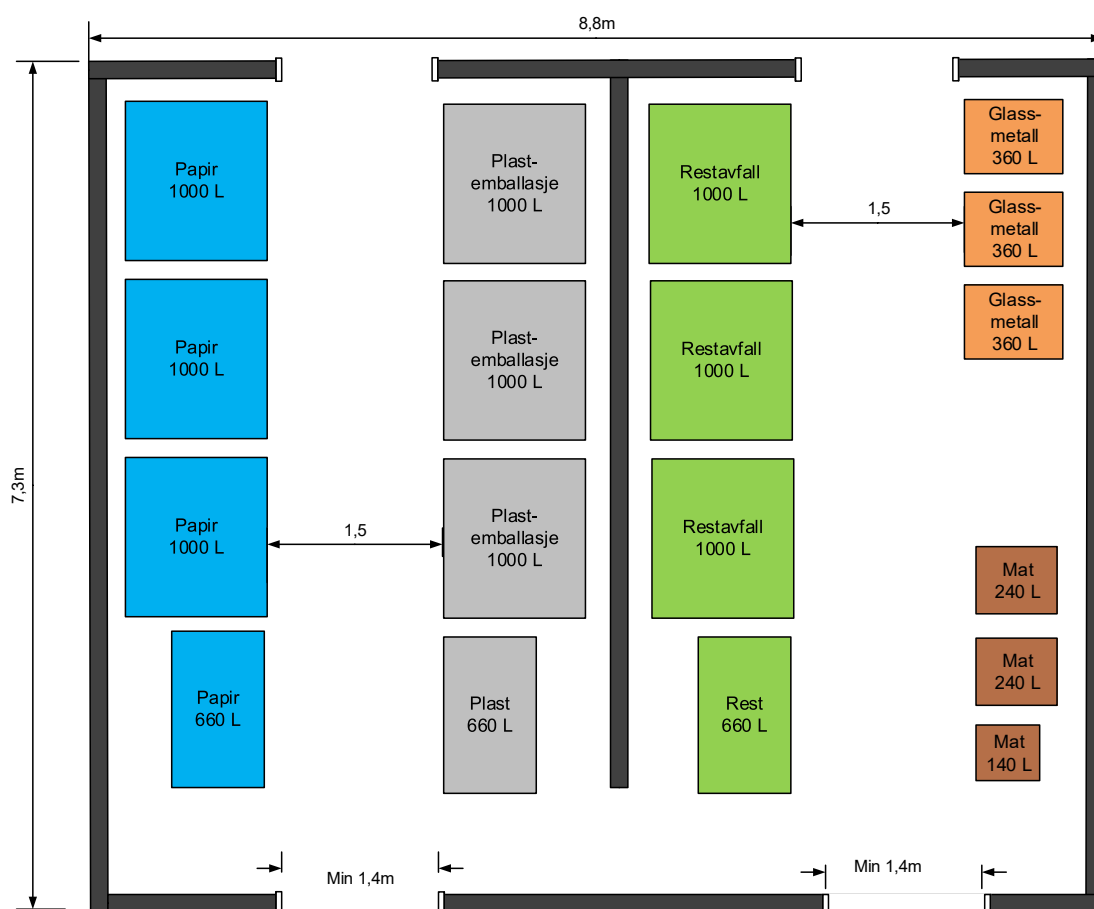
Figur 5-16: Eksempel på planløsning for avfallshus/avfallsrom for 30 husstander
