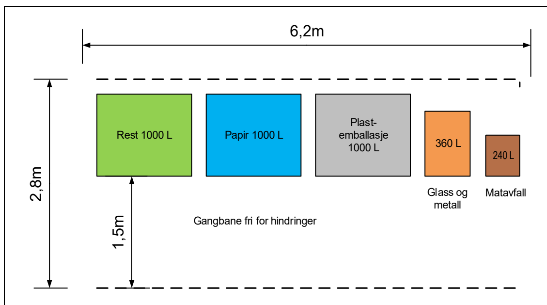
Figur 5-12: Eksempel på planløsning felles standplass for 8 boenheter
