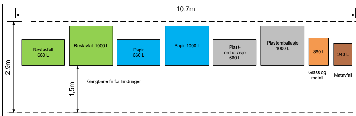
Figur 5-13: Eksempel på planløsning felles standplass for 12 boenheter
