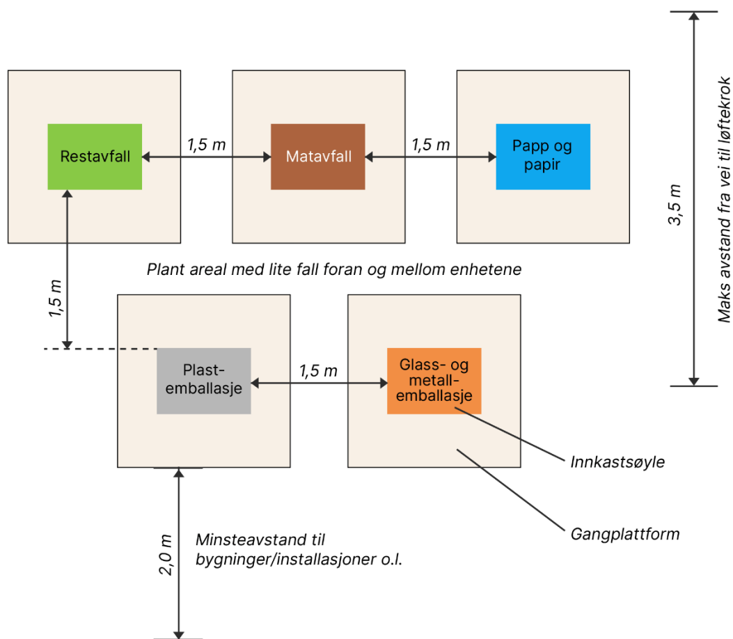
Figur 5-9: Eksempel på arrangement og plassbehov for helt nedgravd løsning for 20 boenheter.
