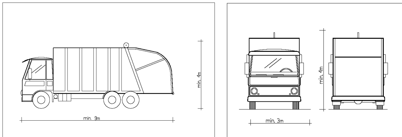
Figur 3-8: Renovasjonsskjøretøy
